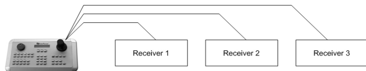
Неправильное подключение шины RS-485
